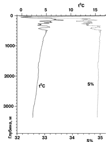
Смешение вод: вертикальное распределение температуры (сплошная линия, верхняя шкала) и солёности (пунктирная линия, нижняя шкала) на полигоне «Титаник» 19 июля 2001 года, по данным гидрофизических зондирований. Видно переслаивание «северных» и «южных» вод ближе к поверхности
