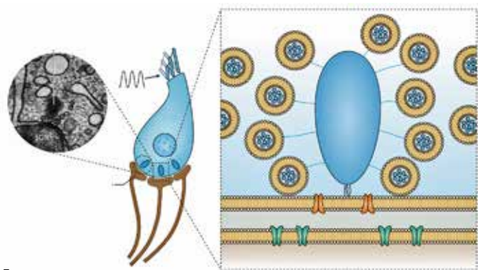
7 Слева электронная микрофотография риббона. В центре схема внутренней волосковой клетки с риббонами на пресинаптической мембране и дендритами нейронов спирального ганглия, образующими синапсы с волосковой клеткой. Справа — риббон с синаптическими везикулами (Nature Reviews Neurology, 2016; doi: 10.1038/nrneurol.2016.10)
