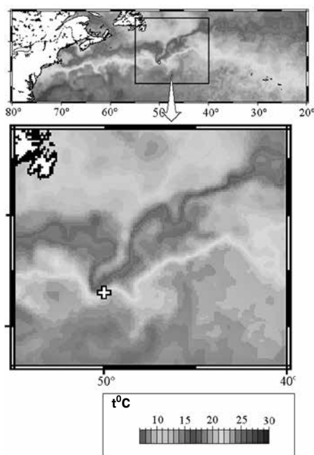
Температура воды на поверхности фронтальной зоны Гольфстрима 19 июля и 22 июля 2001 г., по данным спутниковых измерений; район работ отмечен крестиком. (Использованы суточные карты температуры воды Modular Ocean Data Assimilation System, выставленные в Интернете в свободном доступе Naval Research Laboratory Stennis Space Center.)
