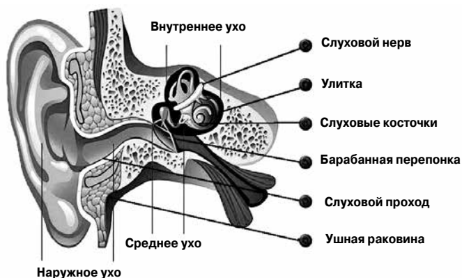
2 Основные отделы уха: наружное, среднее и внутреннее.
