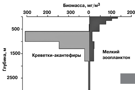
Соотношение биомассы креветок-акантефиров и мелкого зоопланктона в уловах планктонных сетей в столбе воды на полигоне «Титаник» в 1998 году
